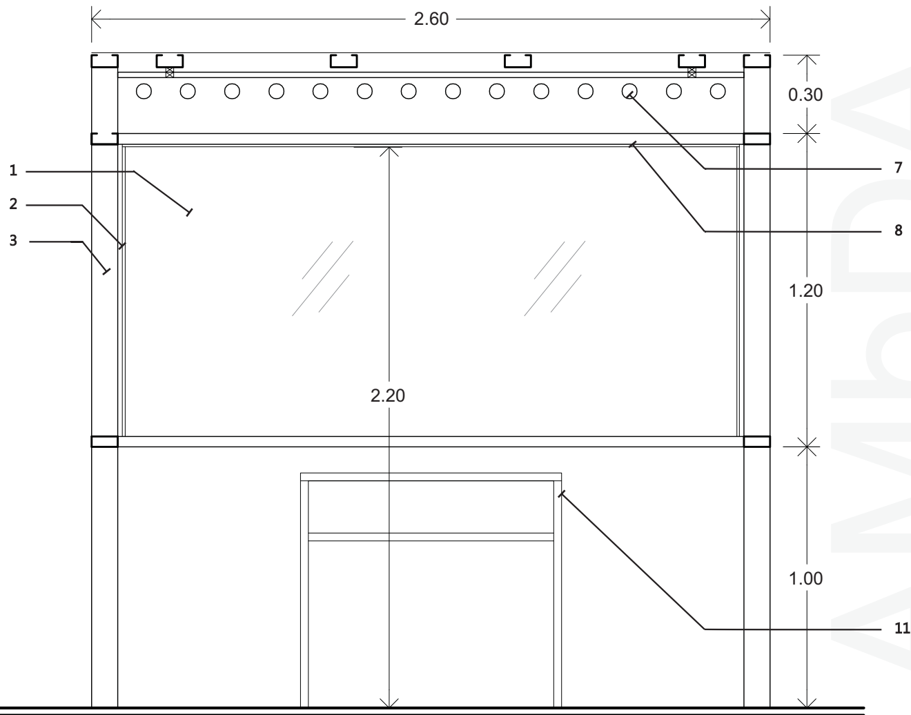
CORTE 1 - 1
